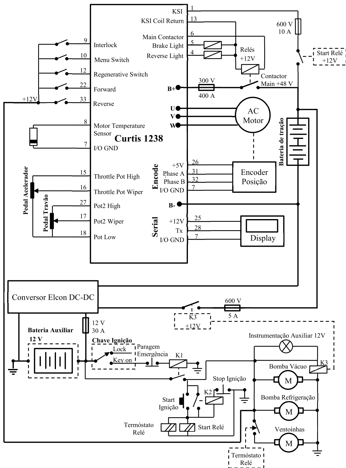
Figura 6-17: Diagrama geral do Power Drive eléctrico.
